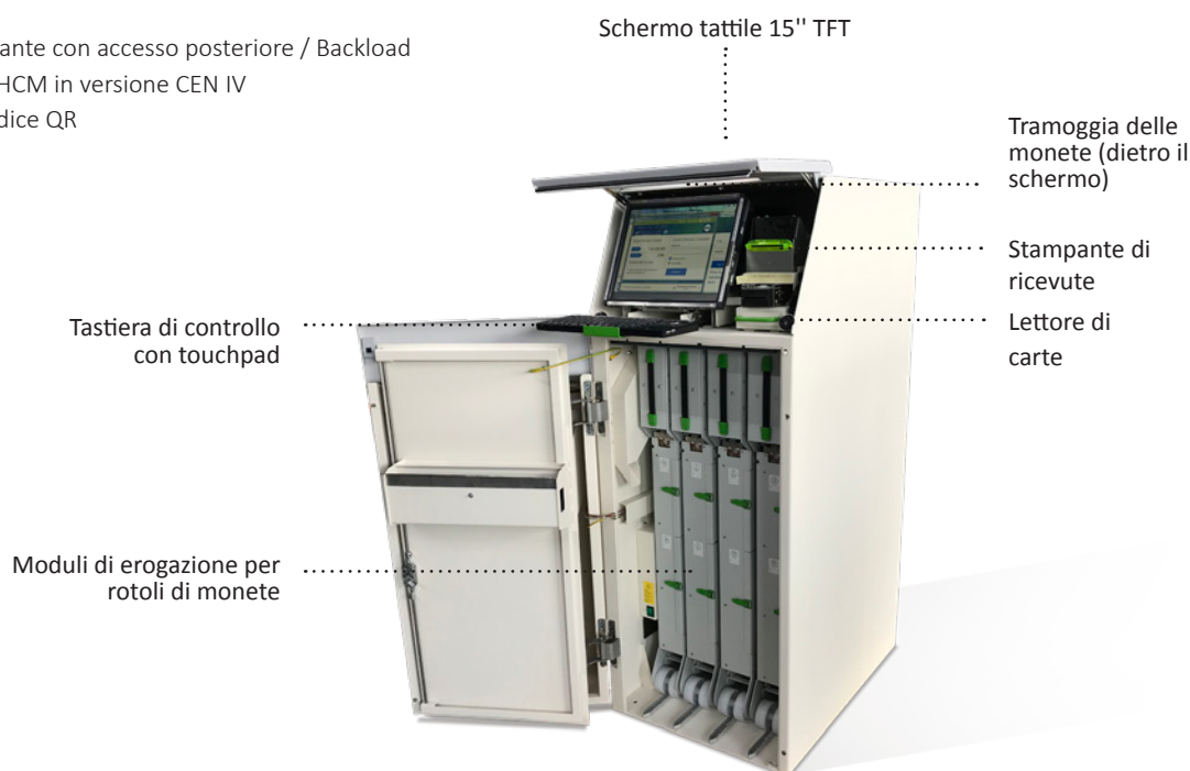
Versione CRC-2610 con accesso frontale ed erogazione di rotoli di monete
